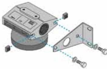
Wandmontagesatz vereinfachte Installation (Größen 9 – 520)
